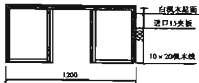
平剖图
