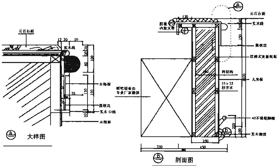
18-105 酒吧台
