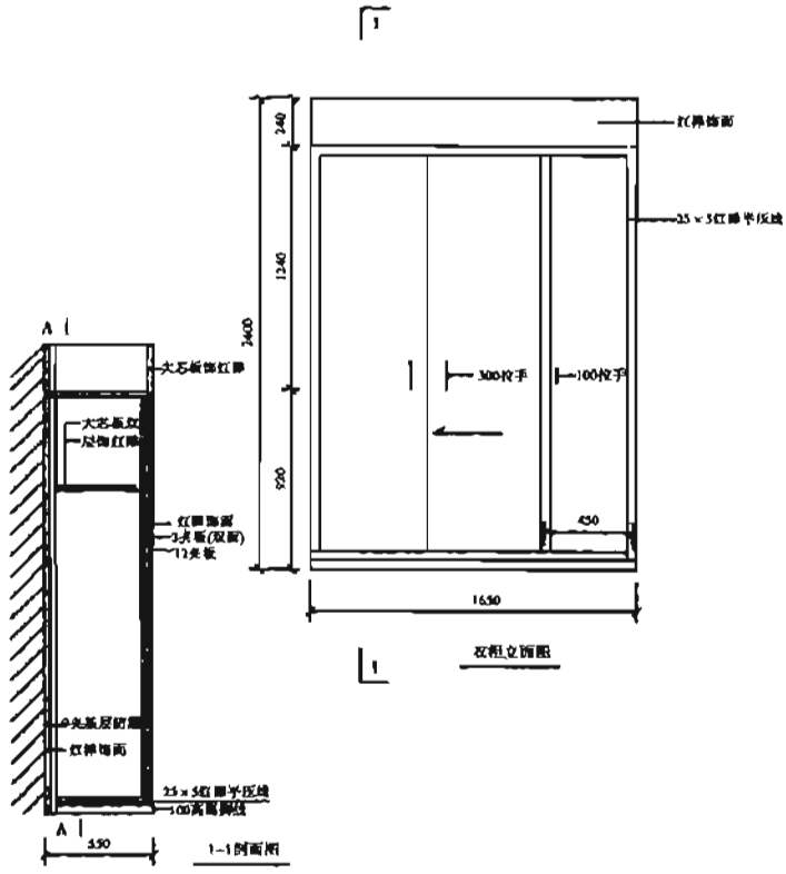
18-113 附墙衣柜
