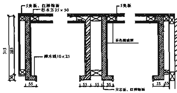
平面图
