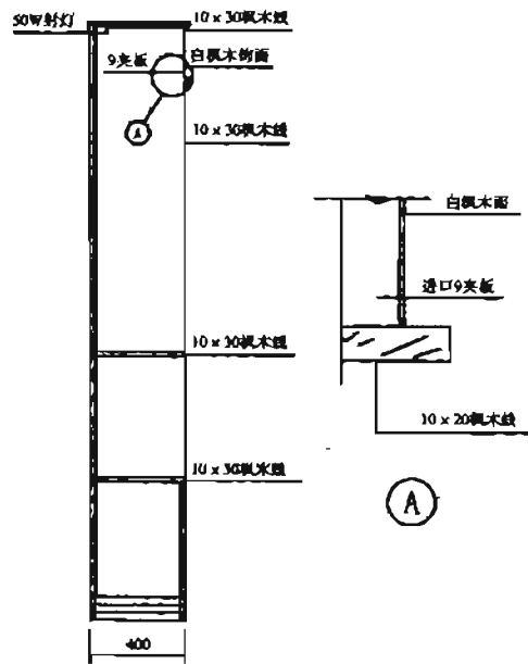
侧剖图
