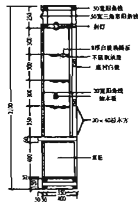
侧立面
