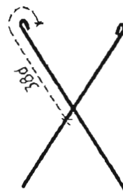
斜筋挑钩计算示意图
