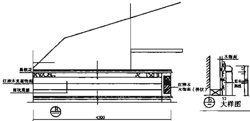
酒吧立面图
