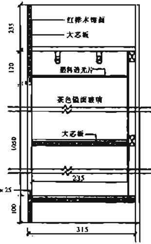
侧立面
