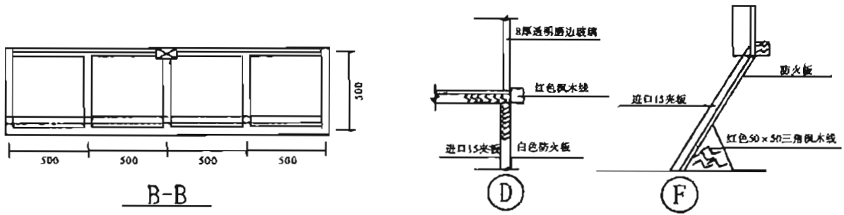
18-94 宝笼1
