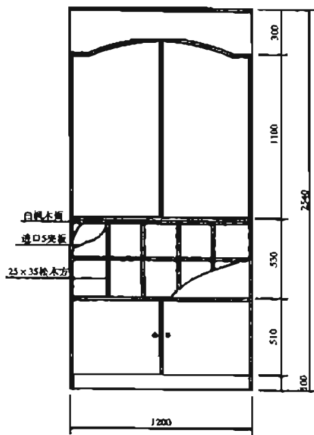
女装精品屋背板架立面图
