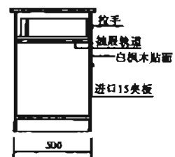
侧剖图
