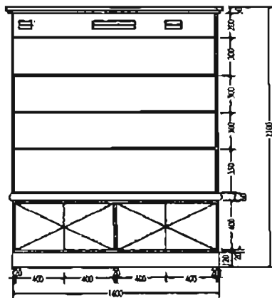
正立面
