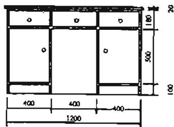
收银台立面图
