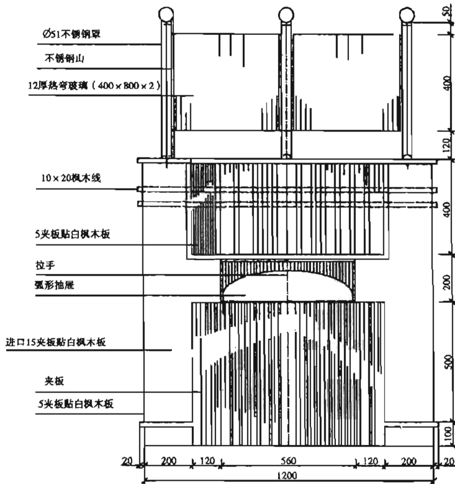
收银台立面
