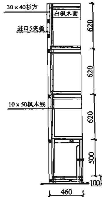
侧剖图
