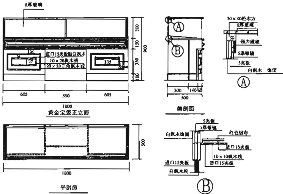
18-95 宝笼2
